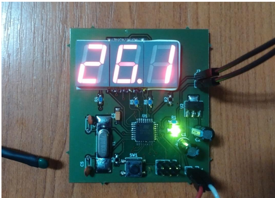
Obrázok 3 - Zrealizované zariadenie
