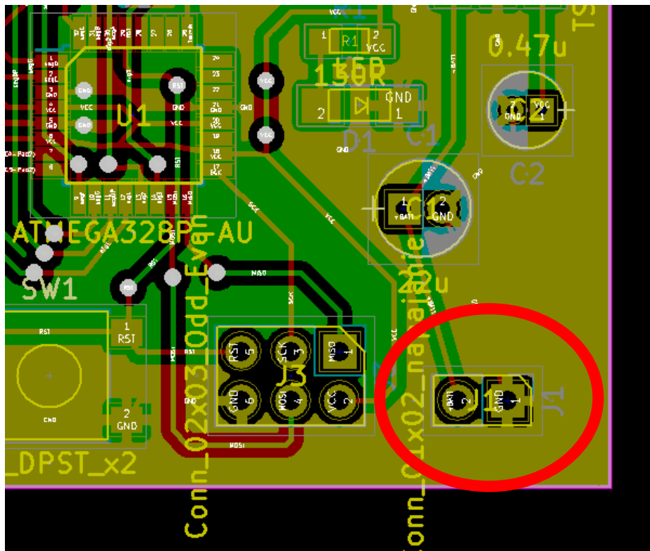
Obrázok 1 - Napájací konektor
